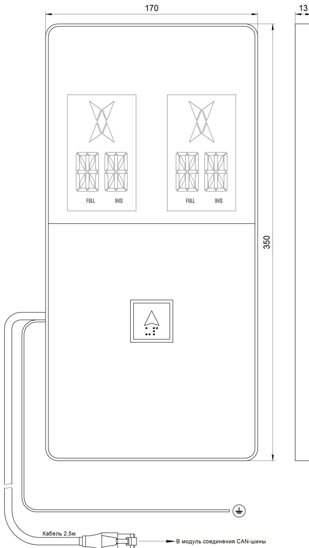
Рис.1 Внешний вид, габаритные и установочные размеры Вызывного поста МАЛАХИТ (жгут RJ45) НШЕК.468381.110
